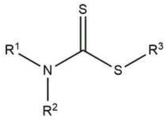
Dithiocarbamates
