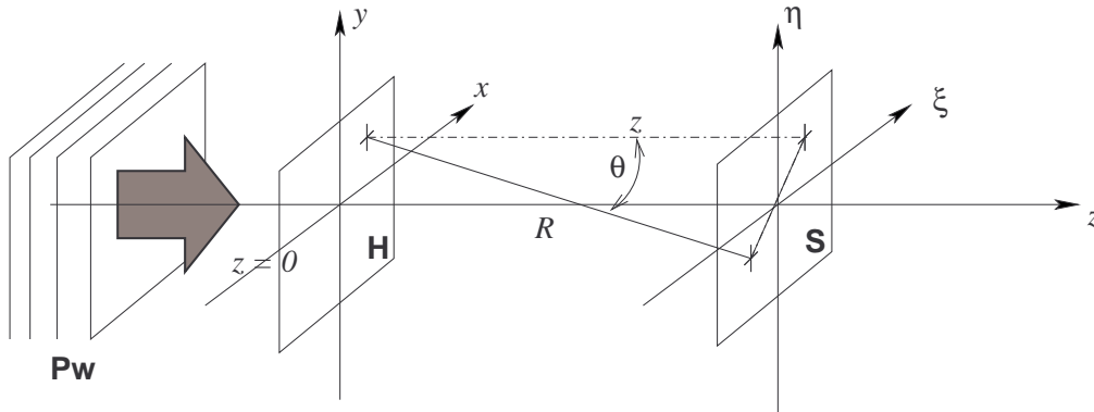
Fig. 2. Configurazione di riferimento per la ricostruzione digitale di un ologramma
