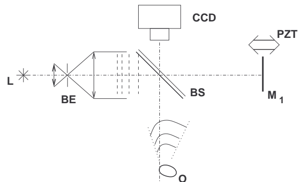
Fig. 3. Setup per olografia digitale
