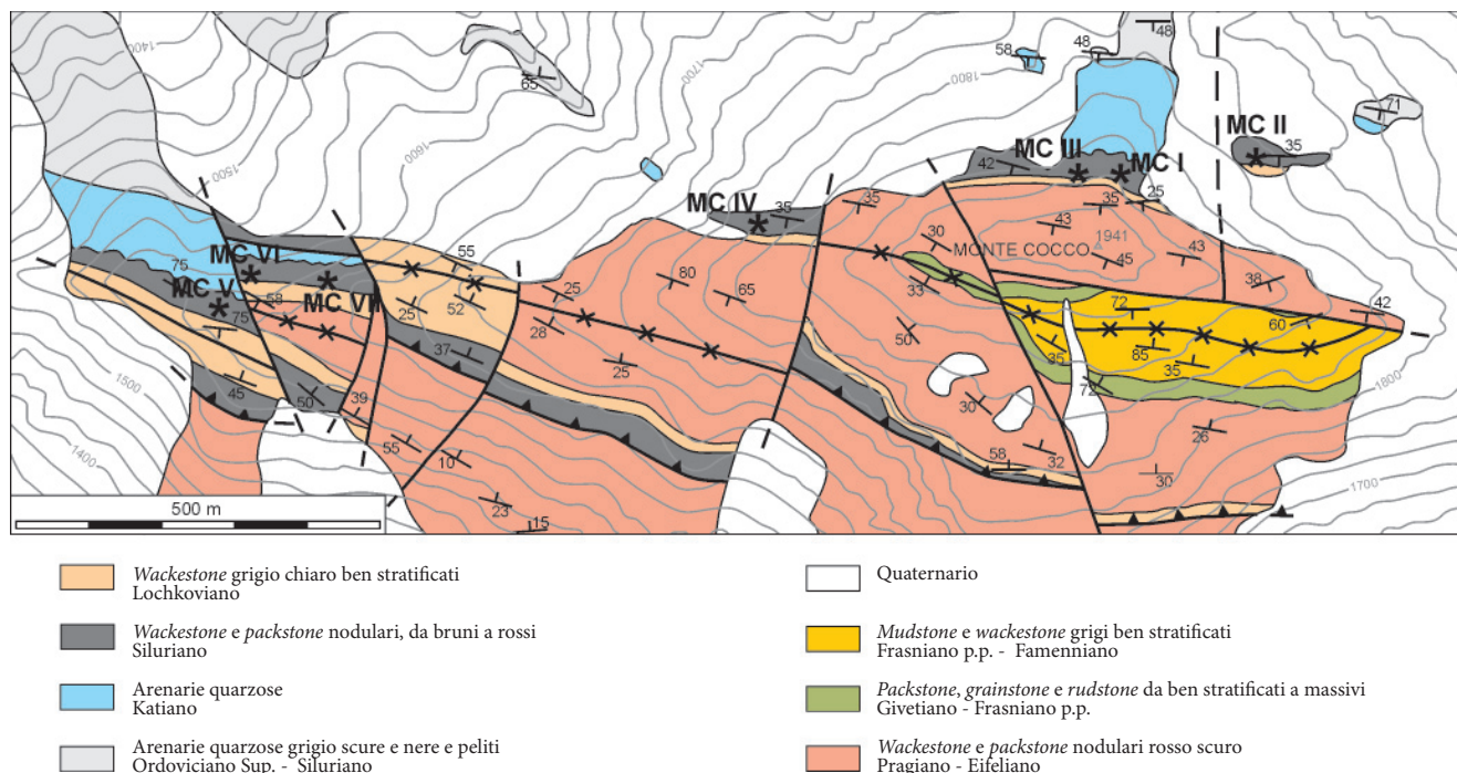
Fig. 2 - Carta geologica dell'area di Monte Cocco con ubicazione delle sezioni stratigrafiche studiate. - Geological map of the Monte Cocco area, with location of the studied stratigraphic sections.
