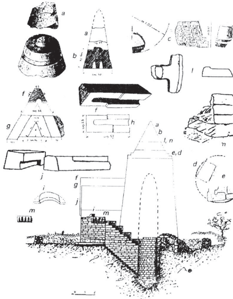
Fig. 1: SERRI – Loc. Santa Vittoria. Sezione della ricostruzione ideale e disegno “esploso” degli elementi architettonici sparsi. Alle lettere posizionate nella sezione (a, b, d-h, m-n) sono fatti corrispondere gli elementi sparsi. C) S. Anastasia, concio conico con modanature; i) Su Tempiesu, archetto monolitico; l) S.Michele-Ittiri, concio a “T” con gibbosità-risega e faccia obliqua (da Contu 1999).
