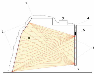
Fig. 12 Schema generale dell'integrazione tra rilievo strumentale e indagine geofisica. Si individua la posizione delle calate G dei geofoni disposti sul paramento, le posizioni dei fori di sondaggio PZ e la posizione delle tomografie CH2, CH6 e CH7. Il tracciato a-a e b-b indica l'area oggetto di indagine con GPR. (Elab. grafica A.Pirinu)
