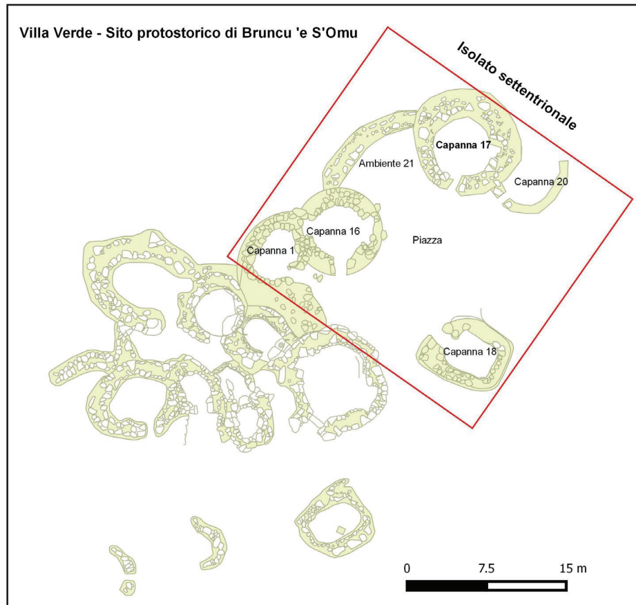
Fig. 1 - Bruncu e' s'Omù, Villa Verde (OR): planimetria generale dell'abitato nuragico e localizzazione dell'isolato settentrionale e delle strutture che lo compongono (con relativa numerazione) (elab. M. Cabras e V. Chergia da Usai, Locci 2008).
