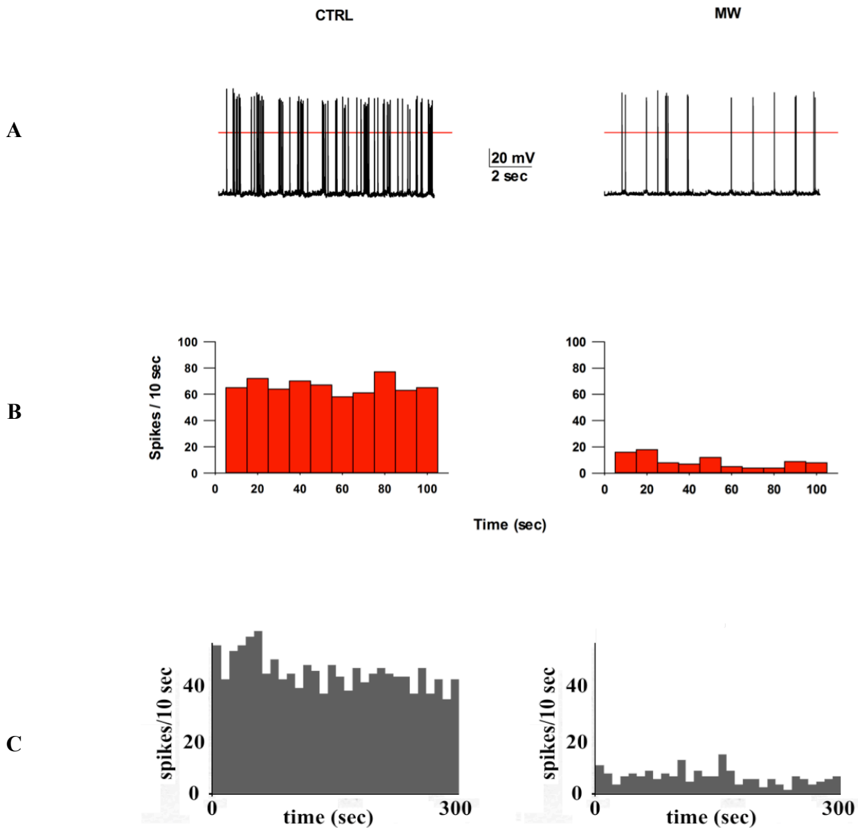
Figura 4 Confronto tra i risultati del modello e i dati sperimentali. A: traccia elettrofisiologica dei primi 10 sec di simulazione, in condizioni di controllo (sinistra) e astinenza da morfina (destra); B: firing frequency del modello; C: dati sperimentali (Diana et al., 1995)
