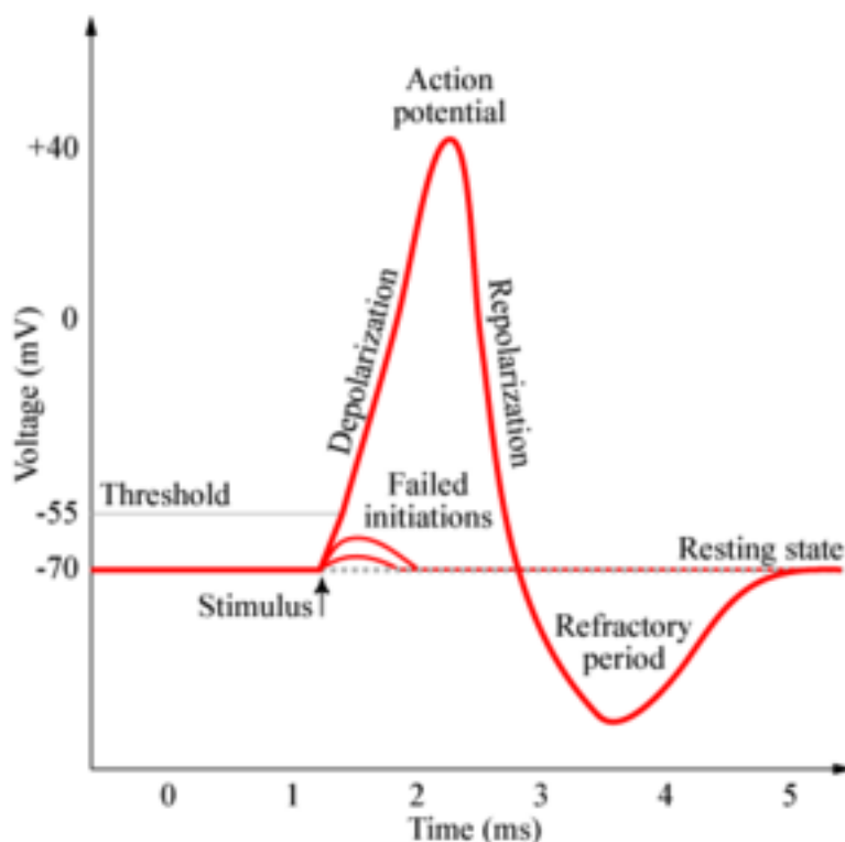
Figura 2 Rappresentazione schematica di un potenziale d'azione.
